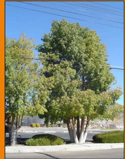
Deux Brachychitons
